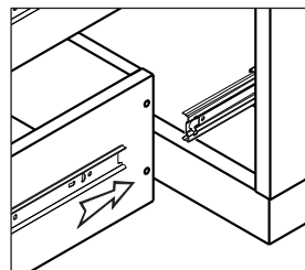
detail 1/detalle 1 drawer placement colocación cajón
